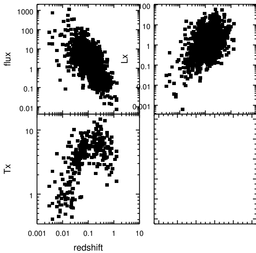
BAX database
