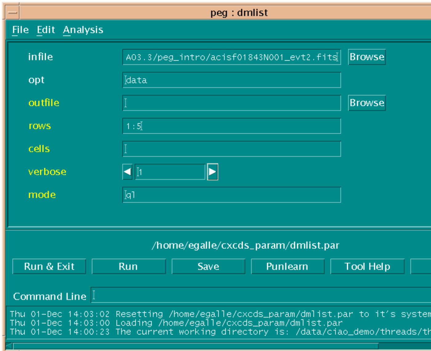
Image 3: Example parameters set
