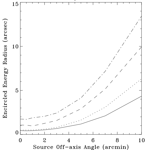
HRMA/ACIS-I1
