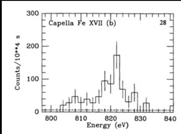
Einstein FPCS
